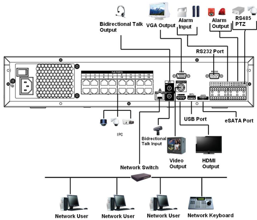
Figura 3-51 Conexión típica
