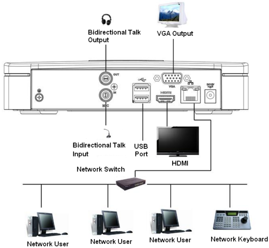
Figura 3-43 Conexión típica
