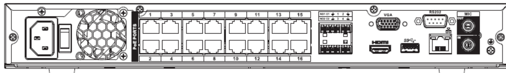
Figura 2-36 Panel trasero
