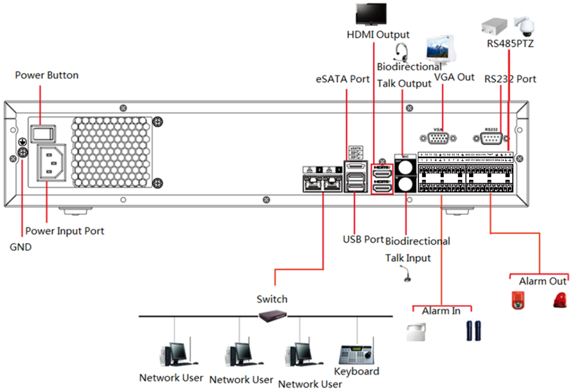
Figura 3-52 Conexión típica
