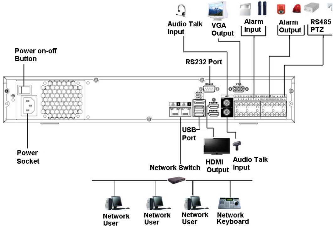
Figura 3-49 Conexión típica
