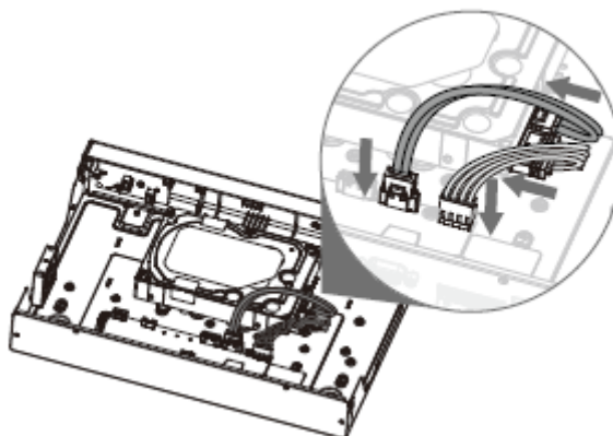
Figura 3-10 Cables de conexión
