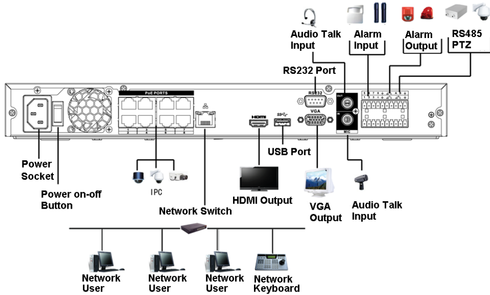
Figura 3-48 Conexión típica
