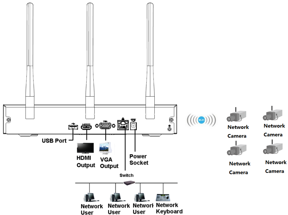
Figura 3-44 Conexión típica
