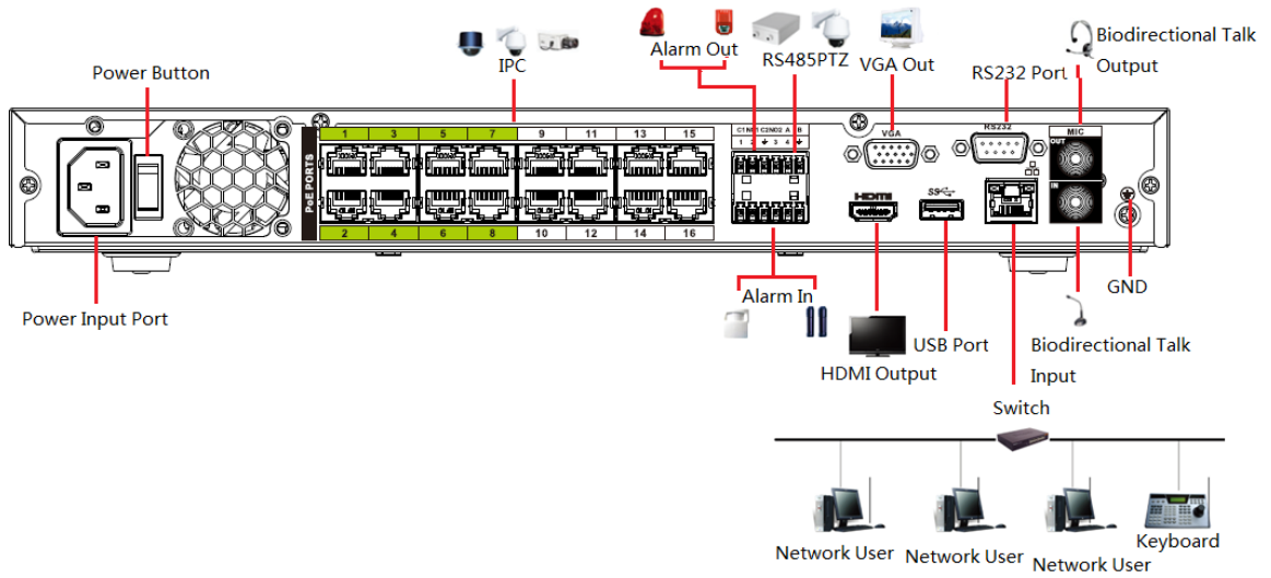
Figura 3-54 Conexión típica
