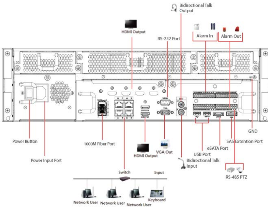
Figura 3-57 Conexión típica
