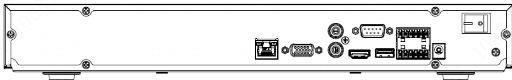
Figura 2-34 Panel trasero
